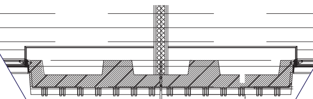
平面図
