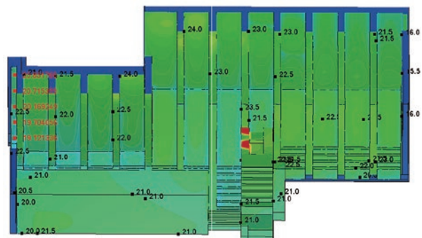
A 通り付近表面温度
