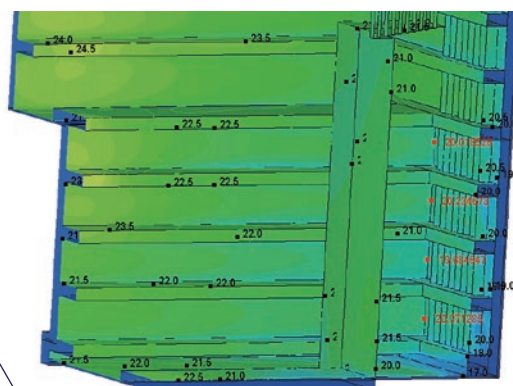
1 通り付近表面温度
